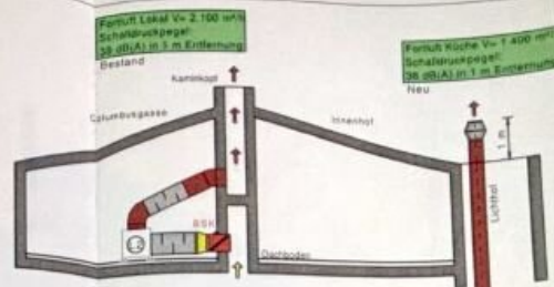
Schnitt Anlage am Dachboden und Fortluft Küche
