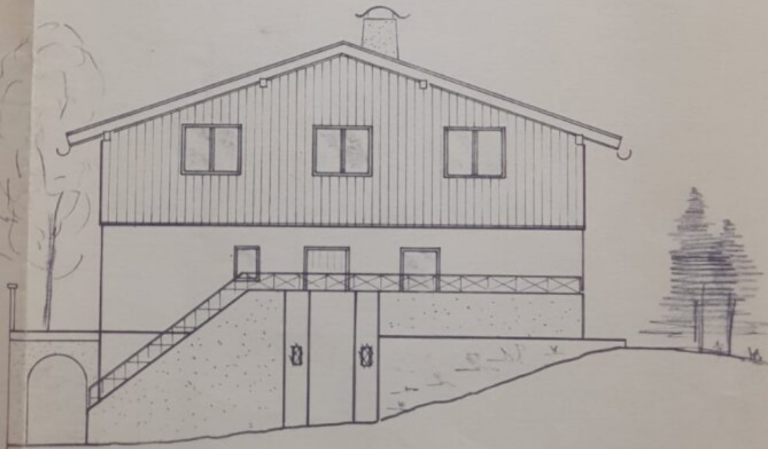
NORD-OST ANSICHT
