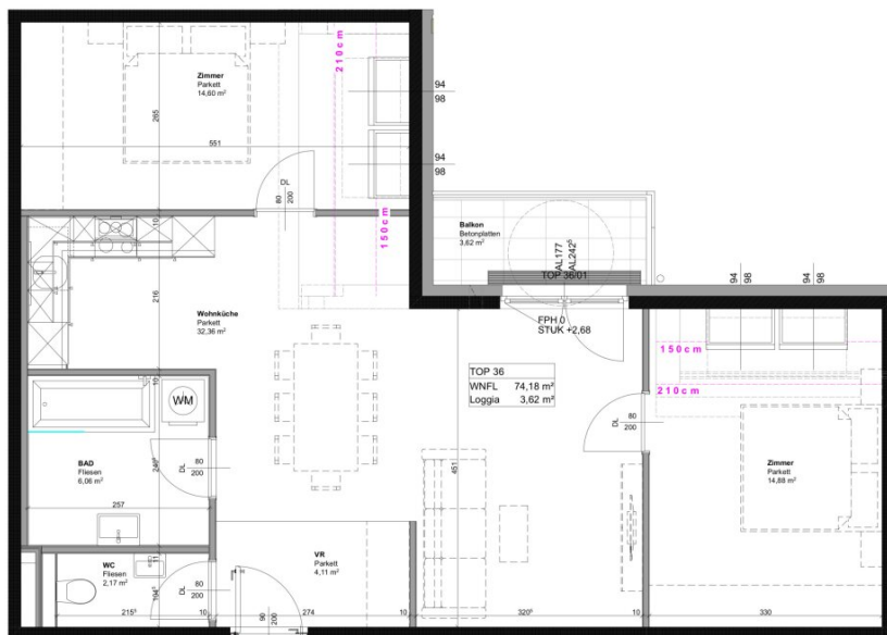
GRUNDRISS 1. DACHGESCHOSS
