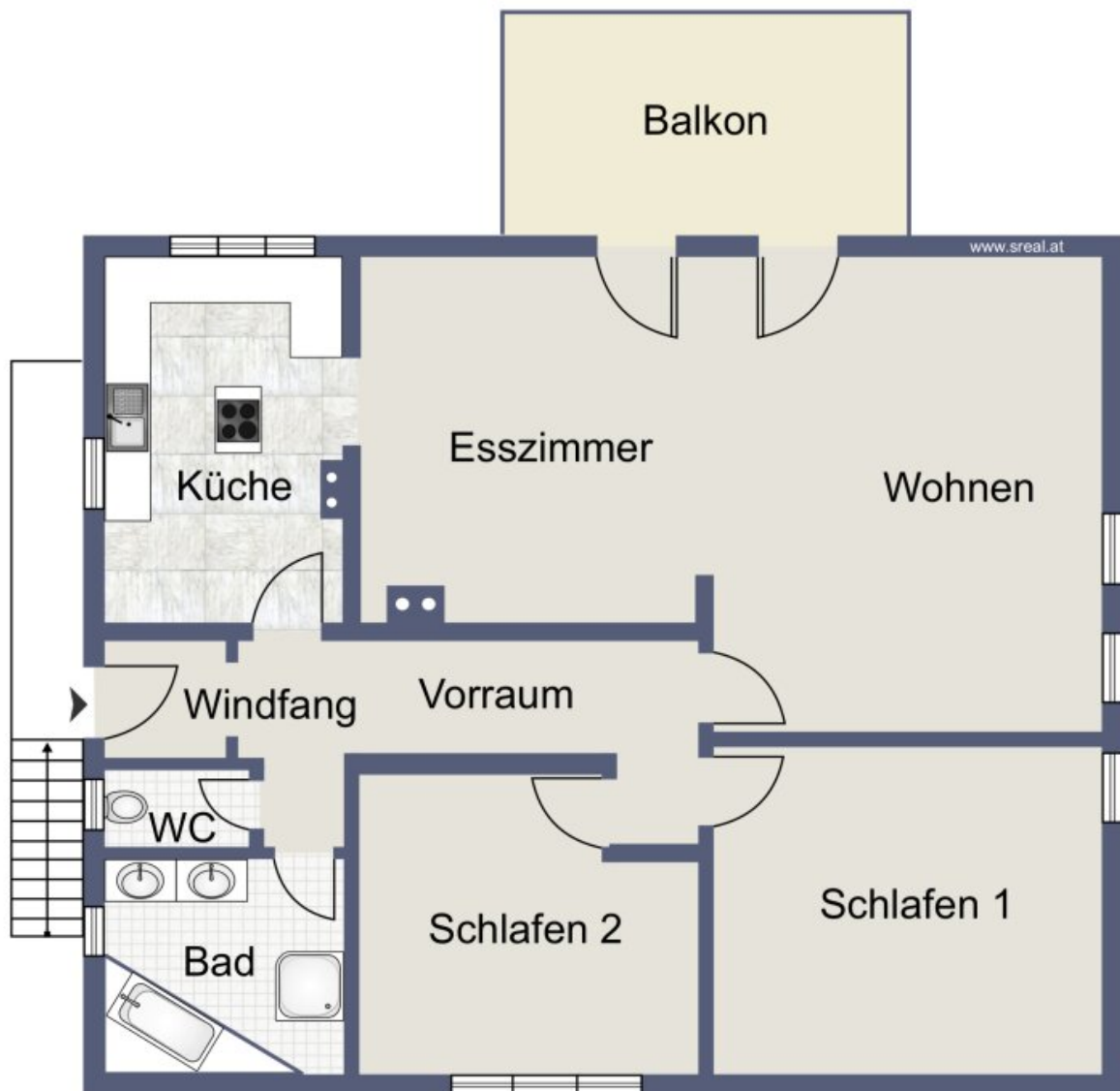
Skizze Obergeschoss Wohnung
