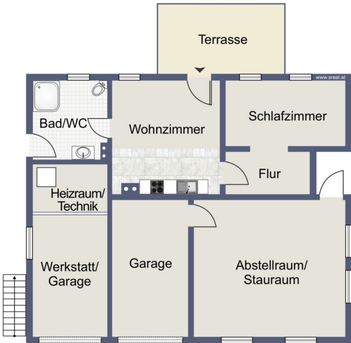
Skizze Erdgeschoss
