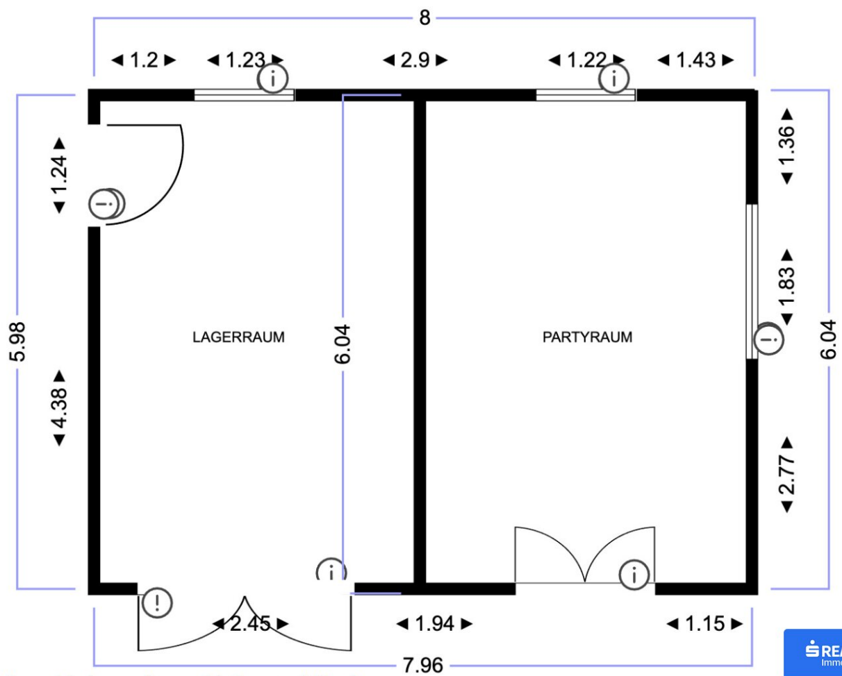
Skizze Erdgeschoss Nebengebäude
