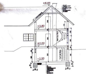
SCHNITT A-A M 1:100
