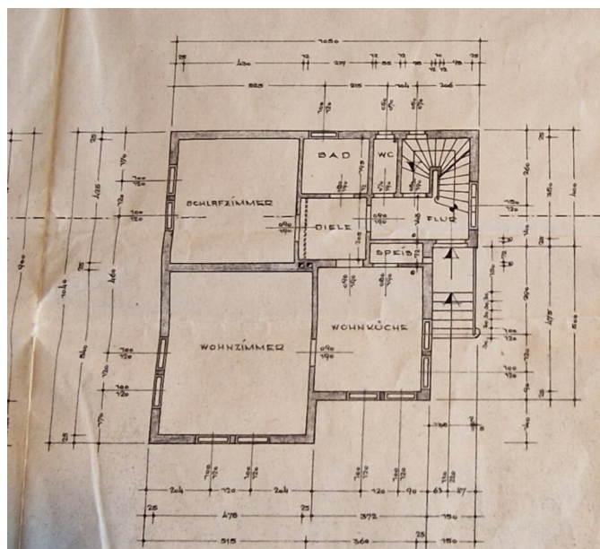
ERDGESCHOSS 1
