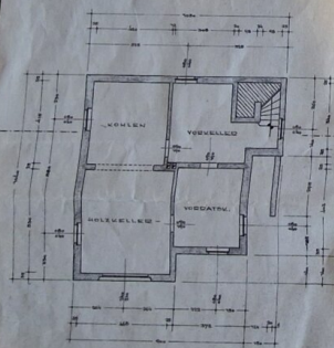
KELLERGECHOSS
