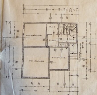
ERDGECHOSS
