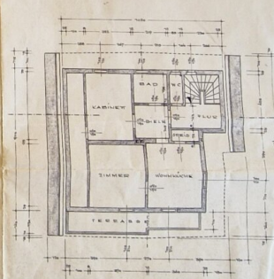
OBERGECHOSS
