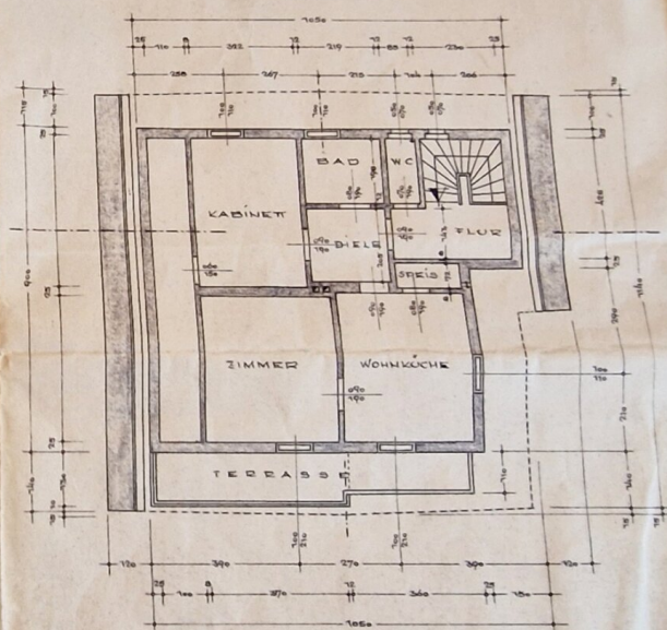
OBERGESCHOSS 1
