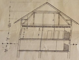
SEHNITT AB
