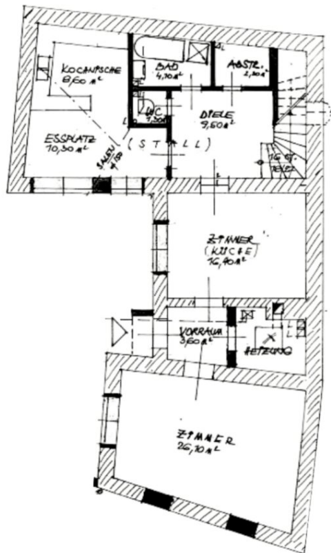
Erdgeschoß
