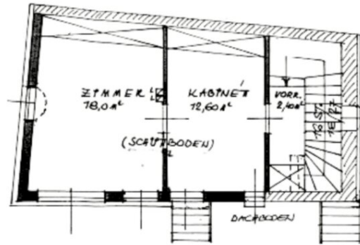
Obergeschoß
