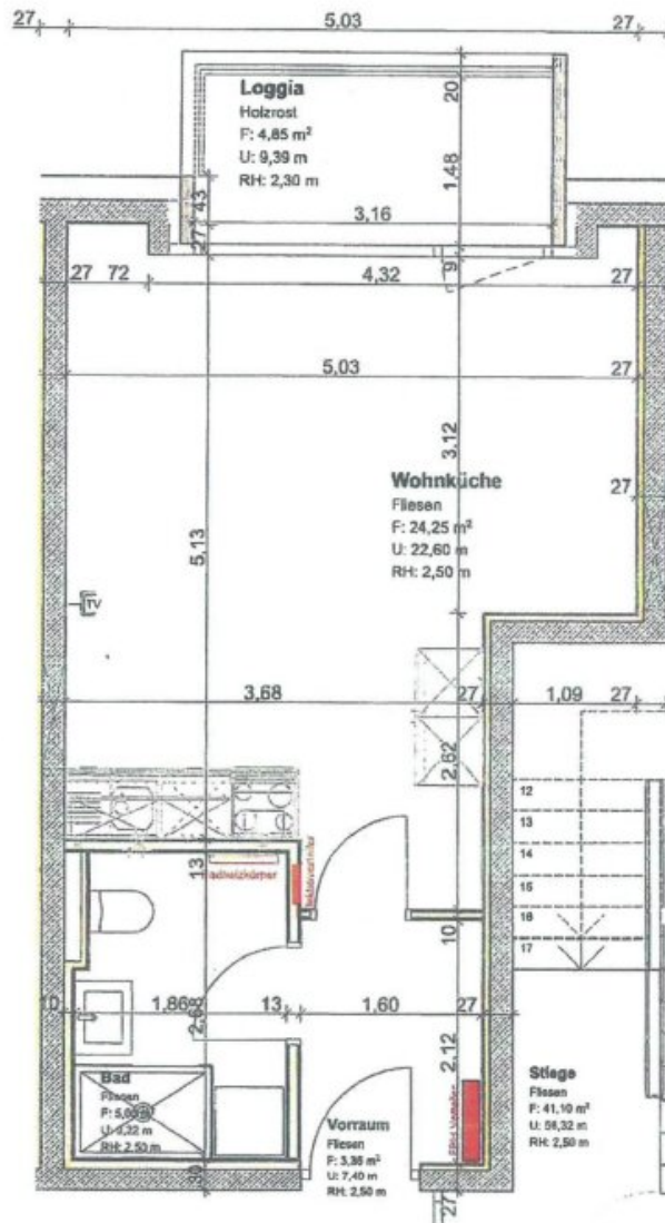
Top 12 1:50 Nutzfläche 32,60 m 2
