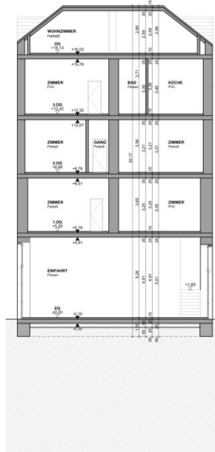
SCHNITT A-A M = 1:100
