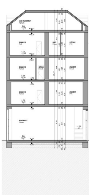
SCHNITT A-A M = 1:100
