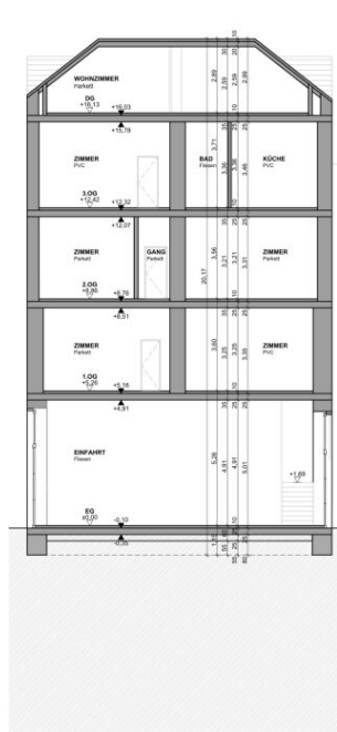
SCHNITT A-A M = 1:100
