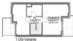
1.OBERGESCHOSS
