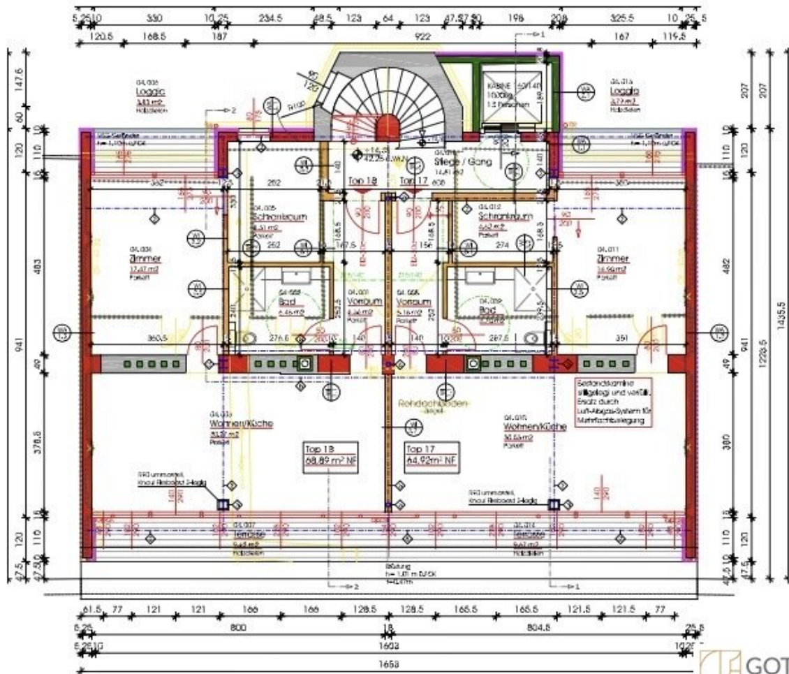
1. DACHGESCHOSS
