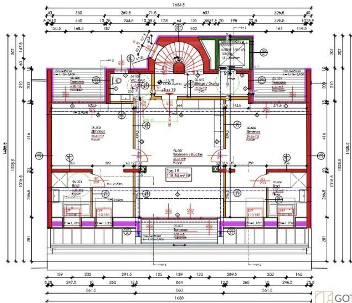
2. DACHGESCHOSS
