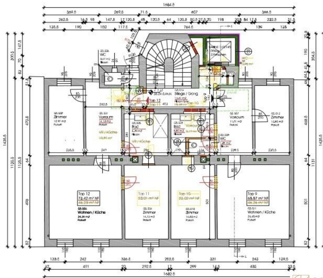
2.OBERGESCHOSS
