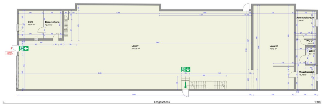
0. Erdgeschoss 1:100
