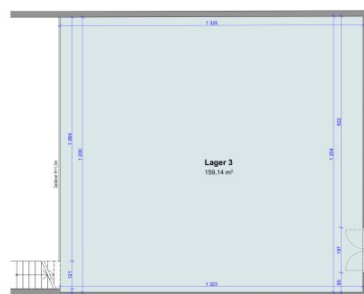
1. Obergeschoss 1:100
