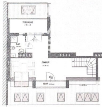
2. Dachgeschoss
