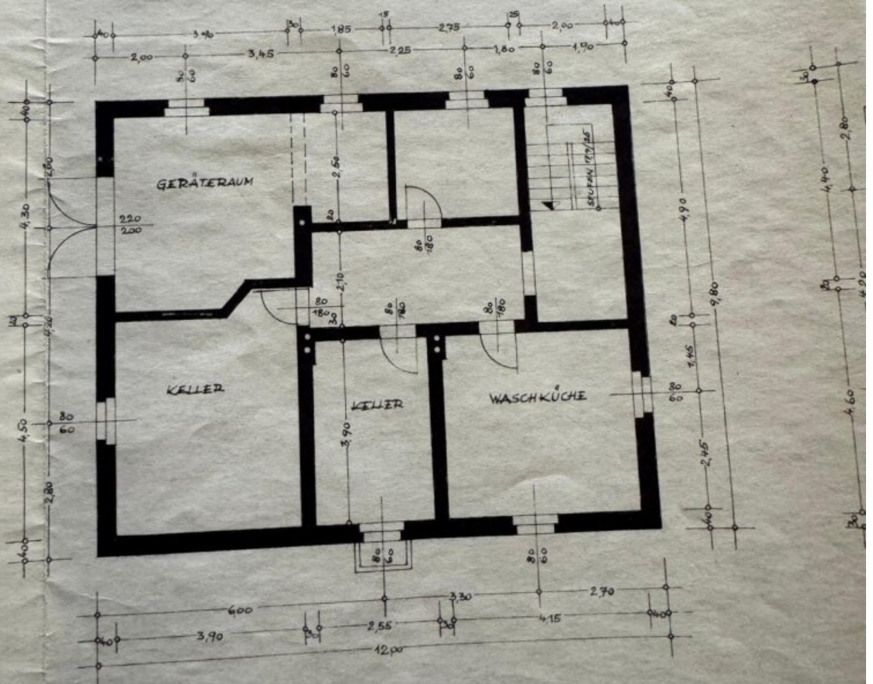
KELLERGRUNDRISS
