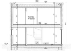
SNITT A-A
