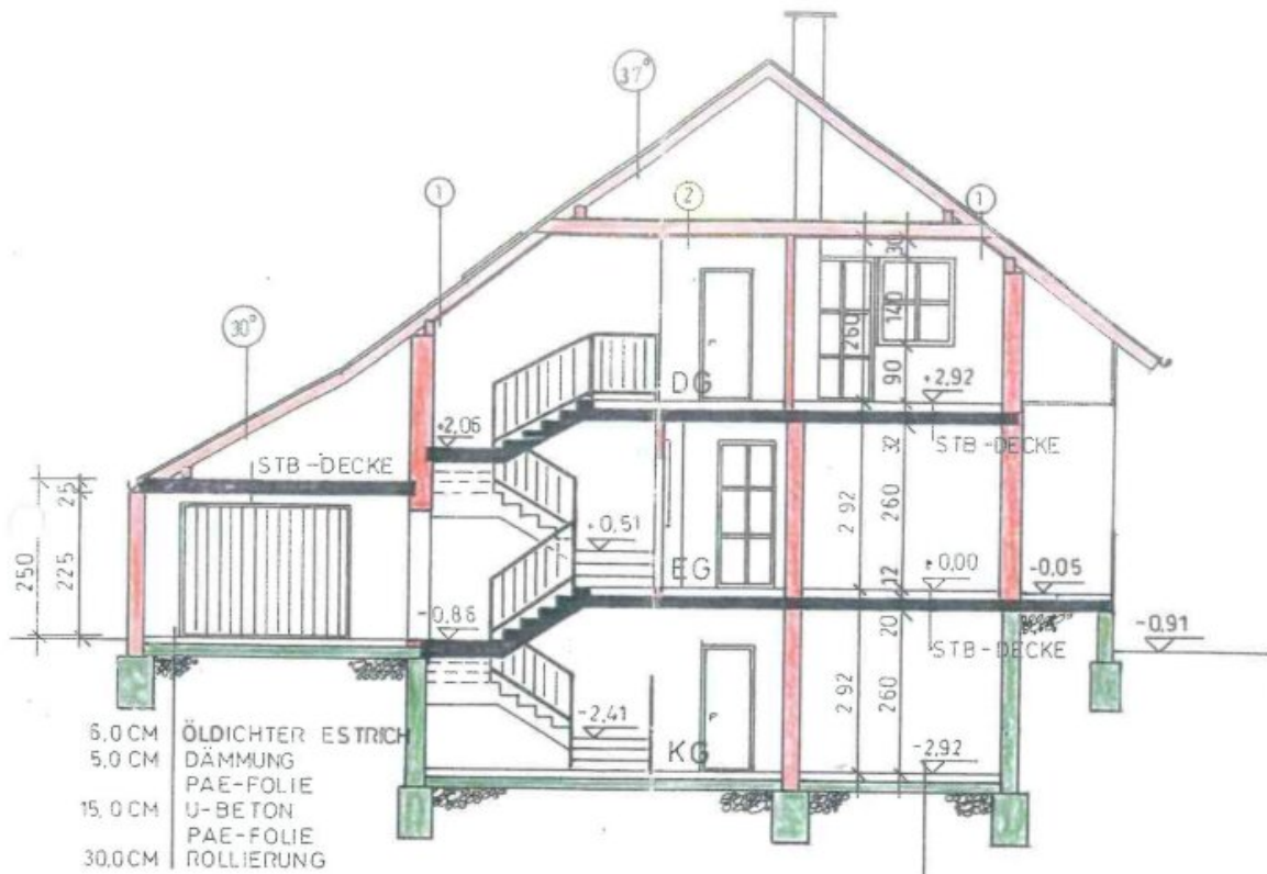
SCHNITT A-A
