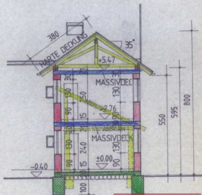
SCHNITT B-B
