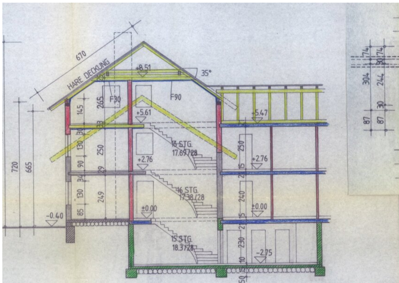
SCHNITT A-A
