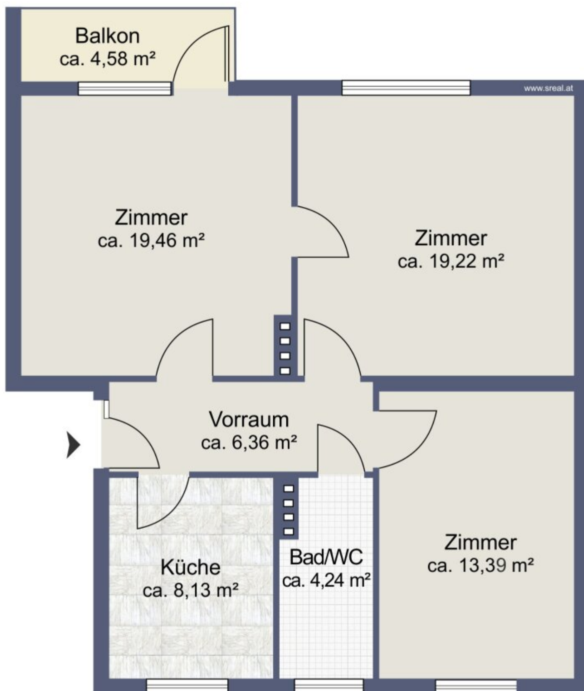
Skizze 2. Obergeschoss
