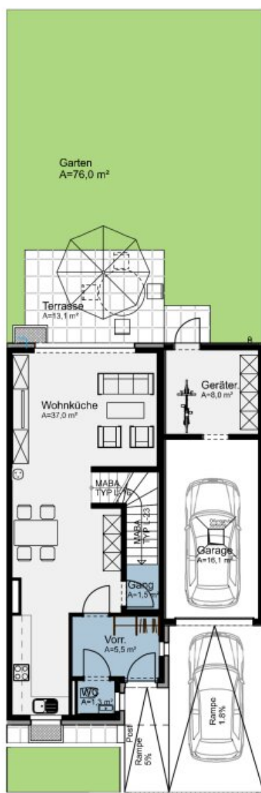
Erdgeschoss
