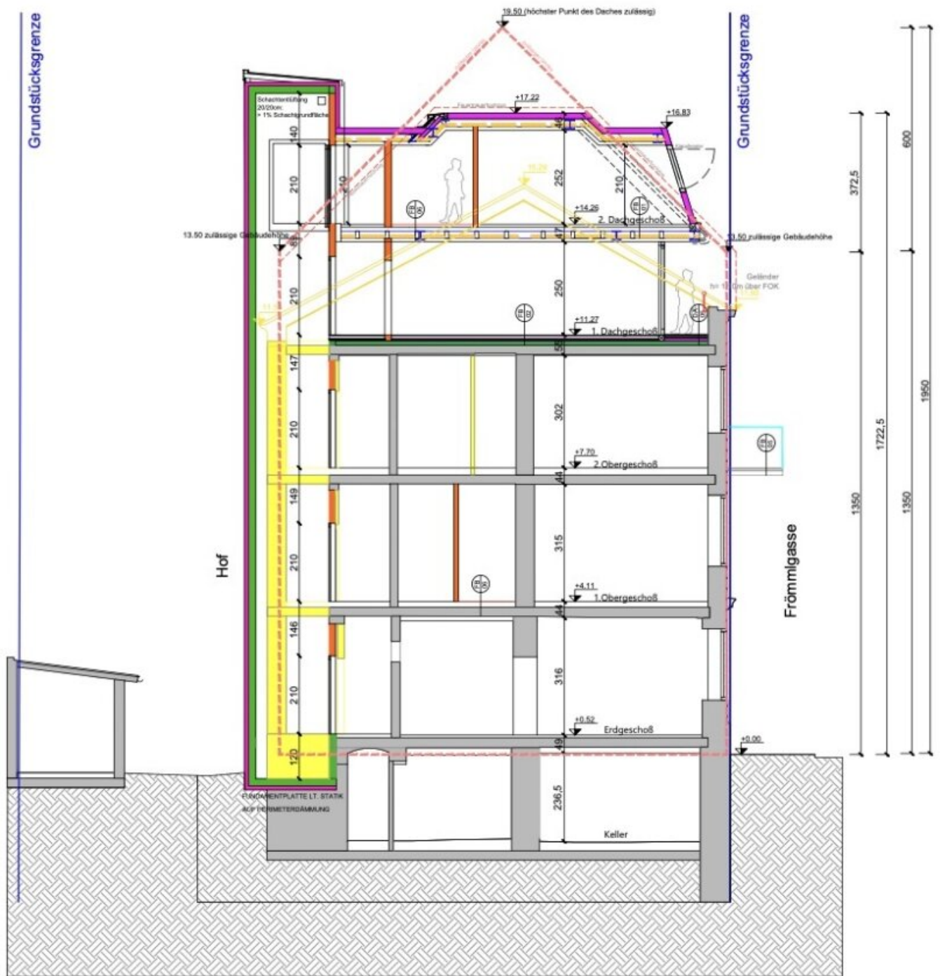
SCHNITT C-C
