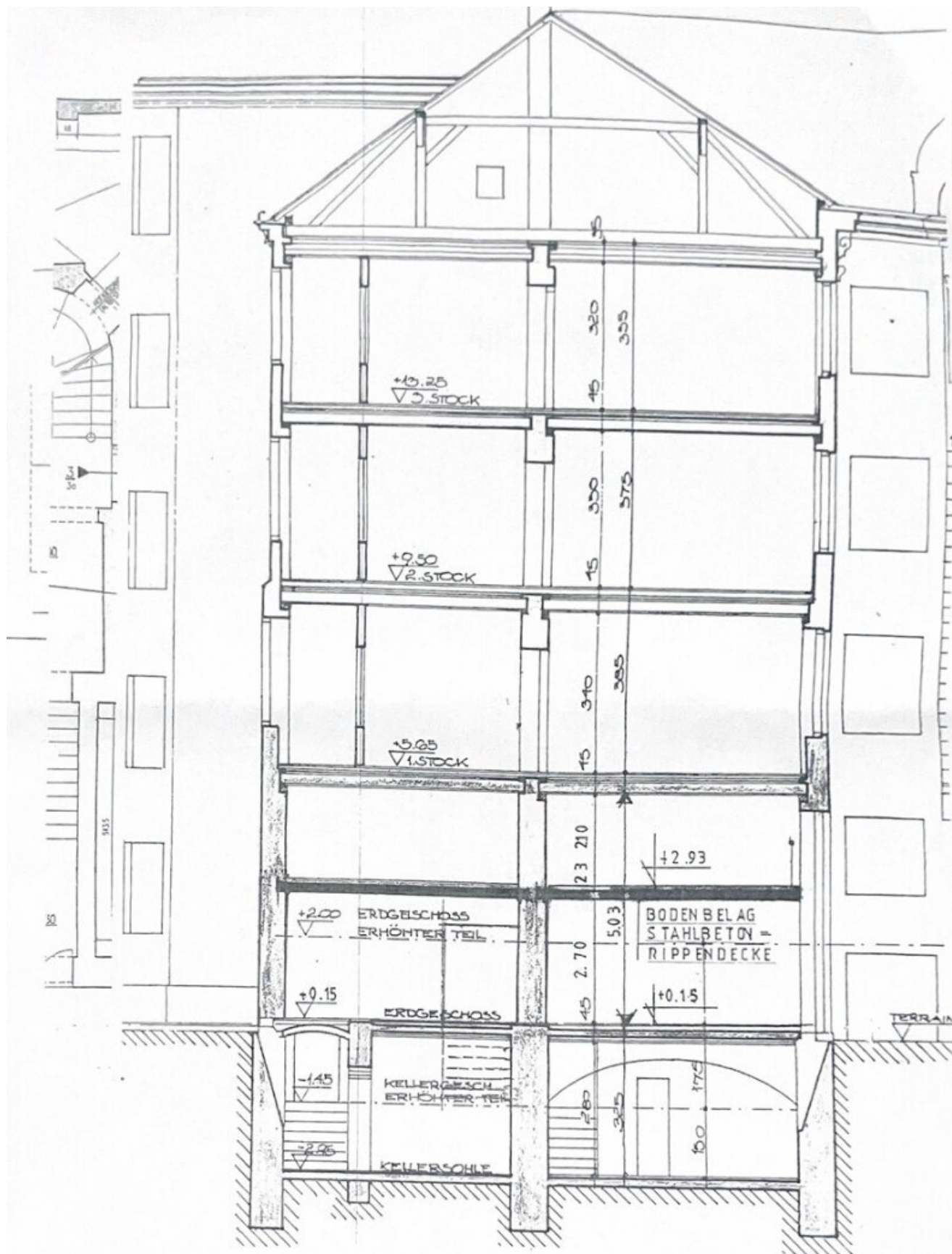
SCHNITT AA
