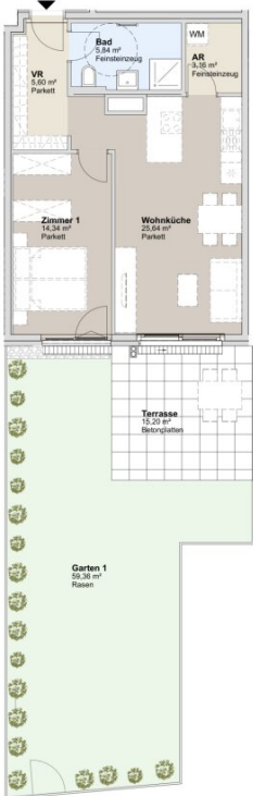
ERDGESCHOSS STRASSENBAUKÖRPER
