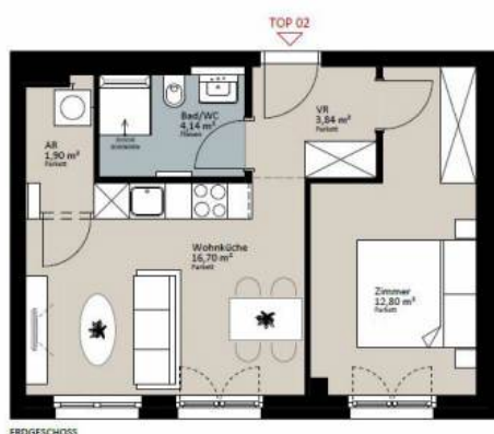
ERDGESCHOSS
