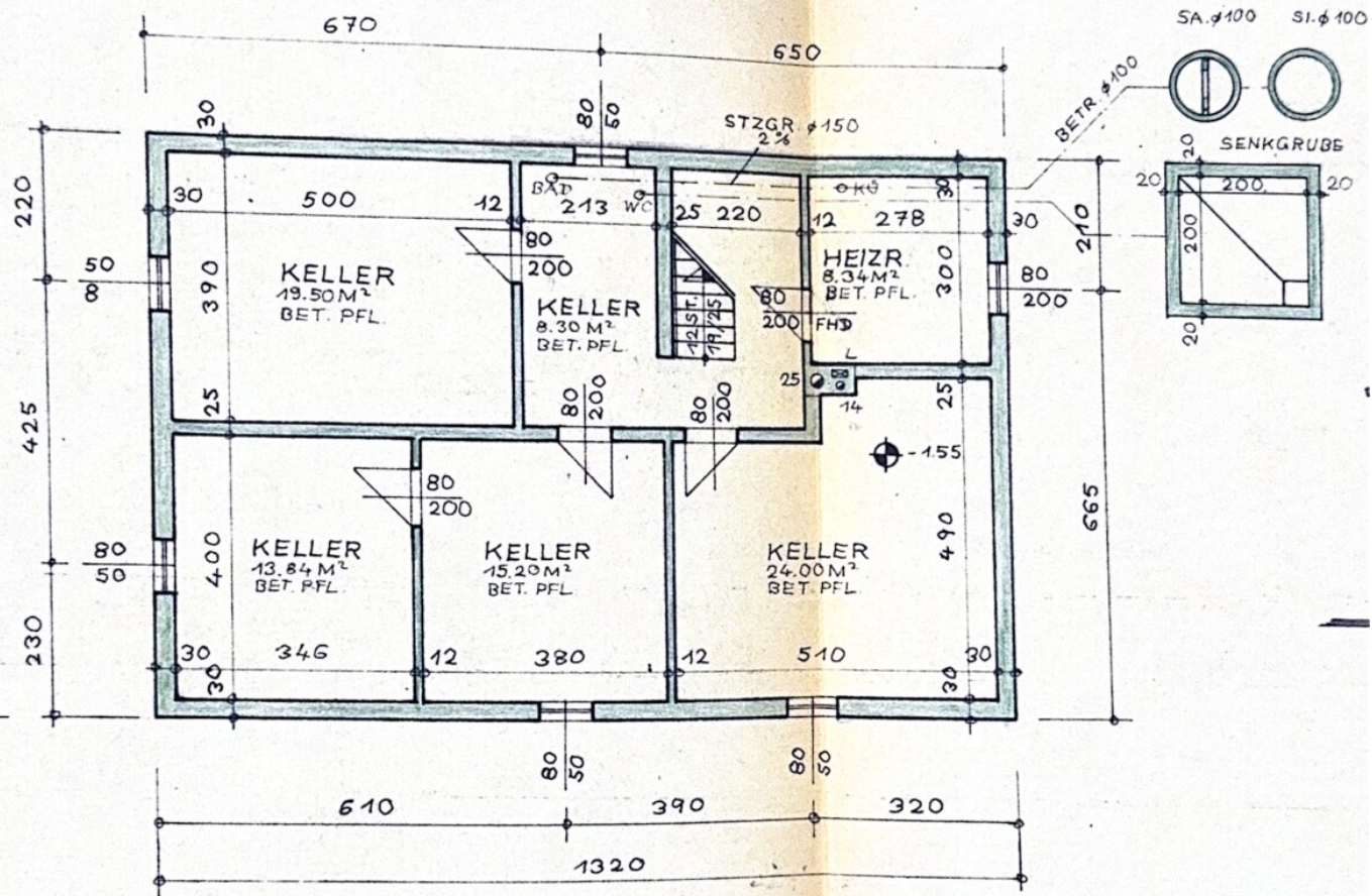
KELLERGEOSCHOSS M=1:100
