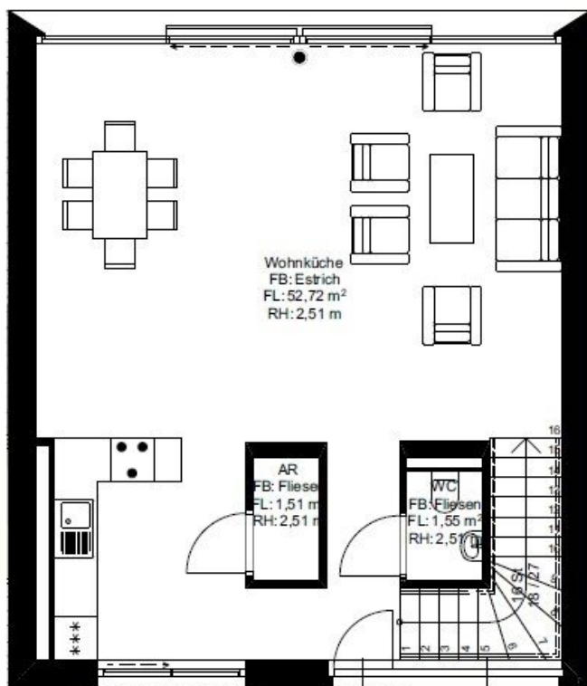
Erdgeschoss 1:100
