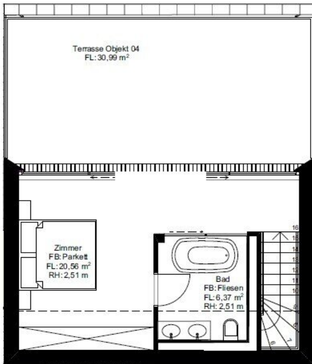
Dachgeschoss 1:100
