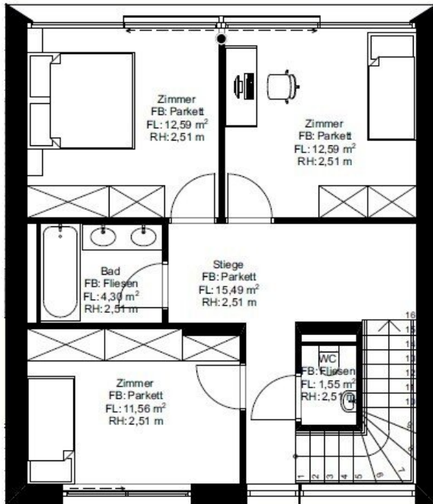
Obergeschoss 1:100
