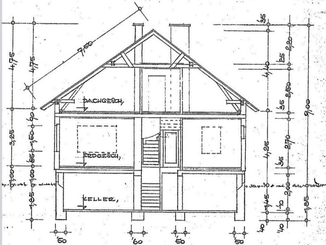
QUER SCHNITT
