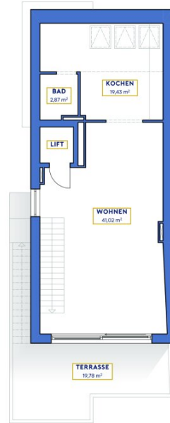
DACHGESCHOSS 1:100
