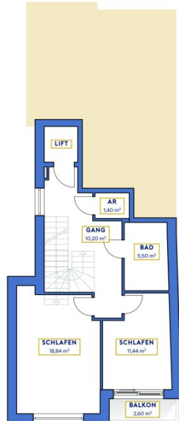
OBERGESCHOSS M 1:100
