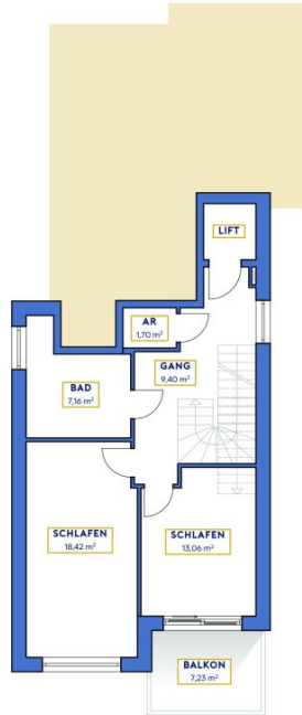
OBERGESCHOSS M 1:100
