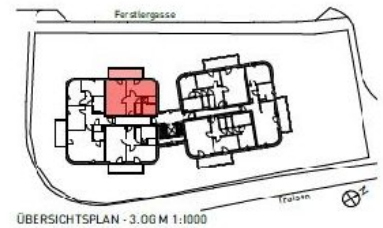
ÜBERSICHTSPLAN - 3.06 M 1:1000
