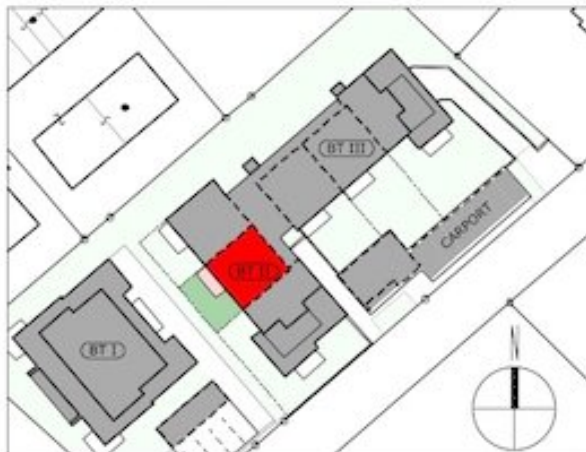
BAUTEIL II - TOP 2: Lageübersicht Wohnung
