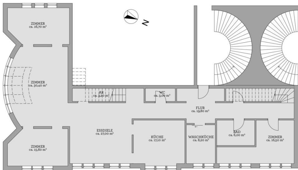
DACHGESCHOSS 1
