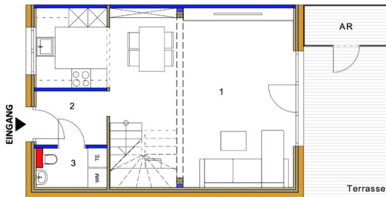
Erdgeschoss M1:75
