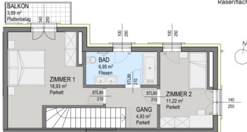
GRUNDRISS: ERDGESCHOSS
