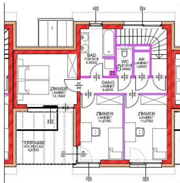
1.OBERGESCHOSS
