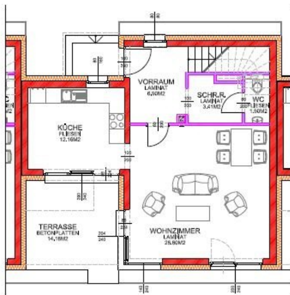
ERDGESCHOSS
