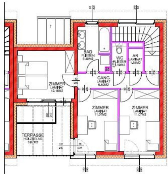
1.OBERGESCHOSS
