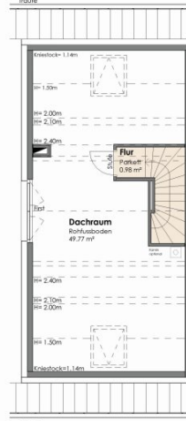
DACHGESCHOSS
