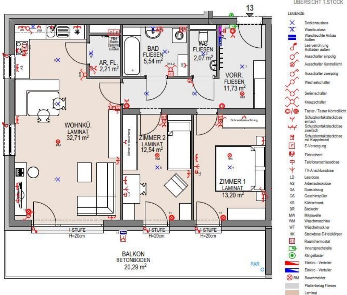
ÜBERSICHT 1.STOCK
