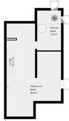
Kellergeschoss
