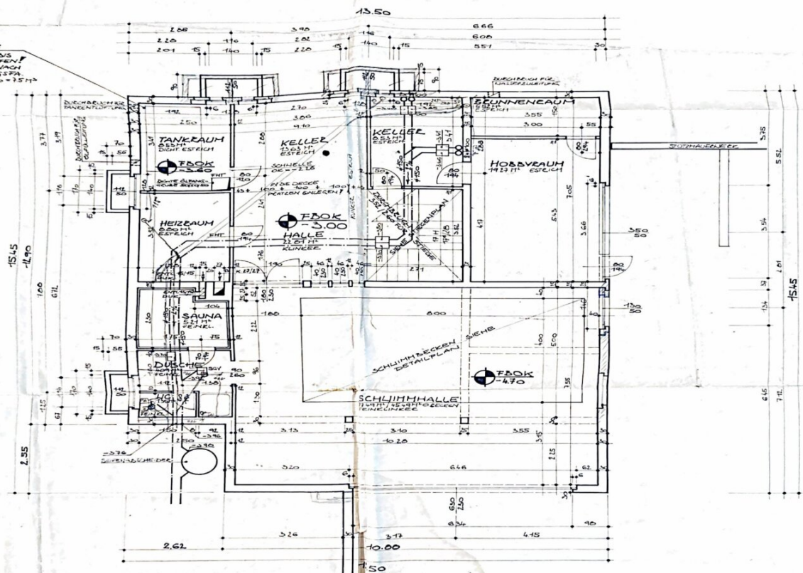
UNTERGESCHOSS M1:50
