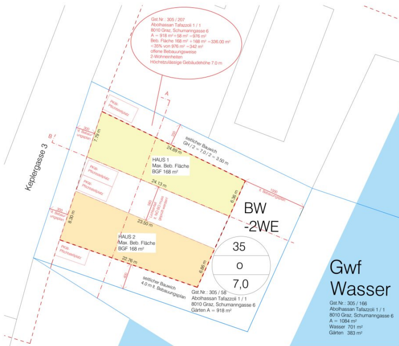
LAGEPLAN M 1:250
