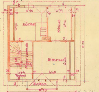
Grundriss Dachstuhl
