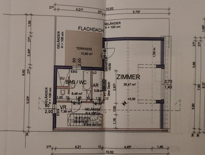
GRUNDRISS DG
