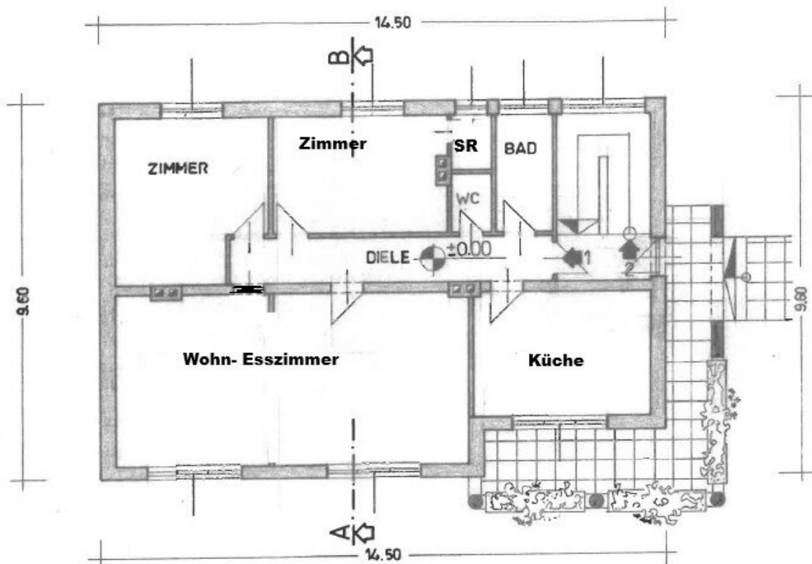
GRUNDRISS - ERDGESCHOSS (BESTAND)
