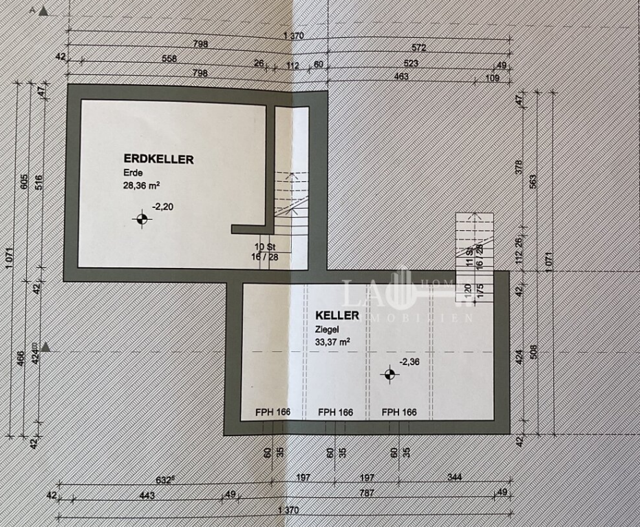
GRUNDRISS KG
