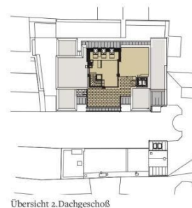
Übersicht 2. Dachgeschoß
