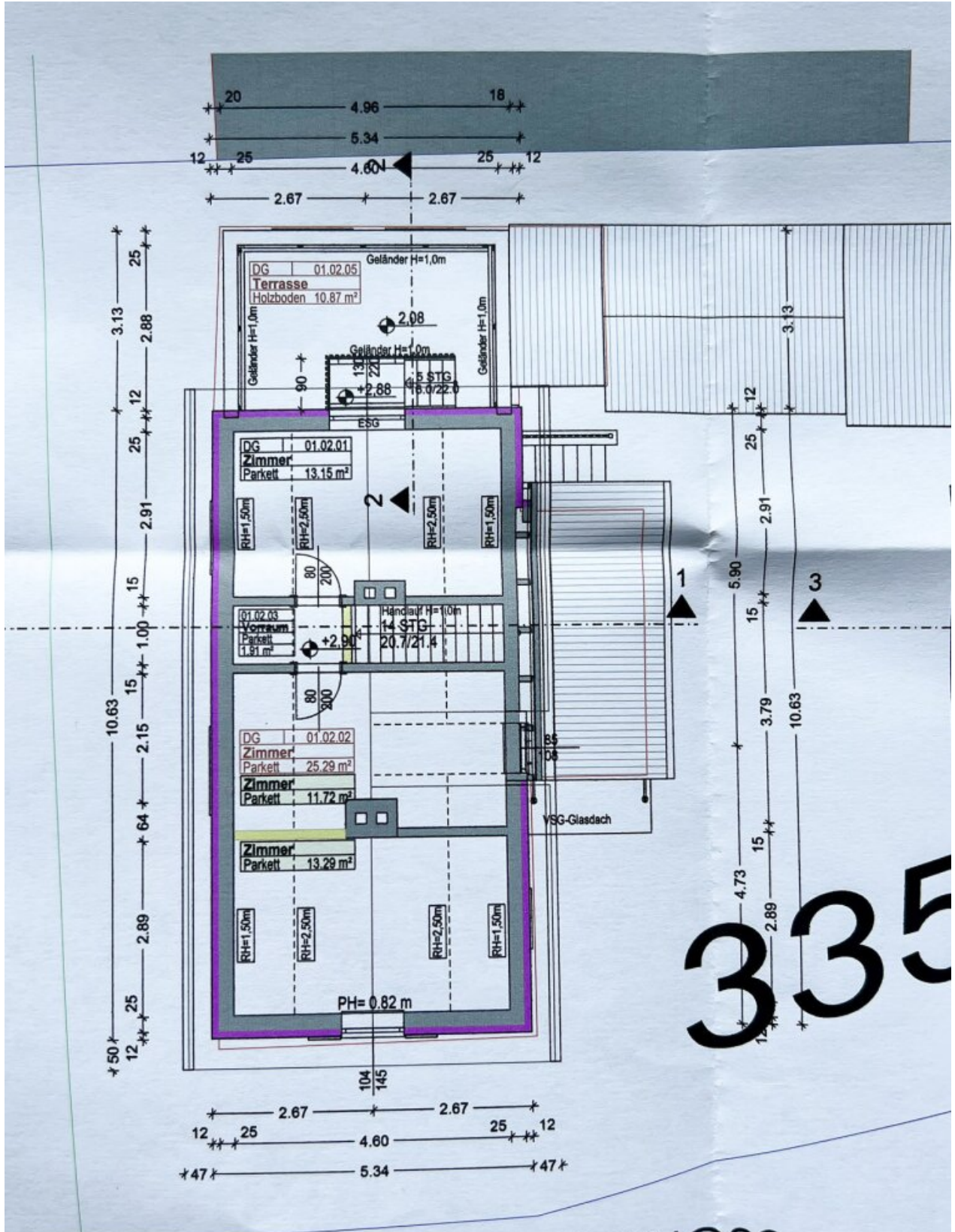
GRUNDRISS DACHGESCHOSS
