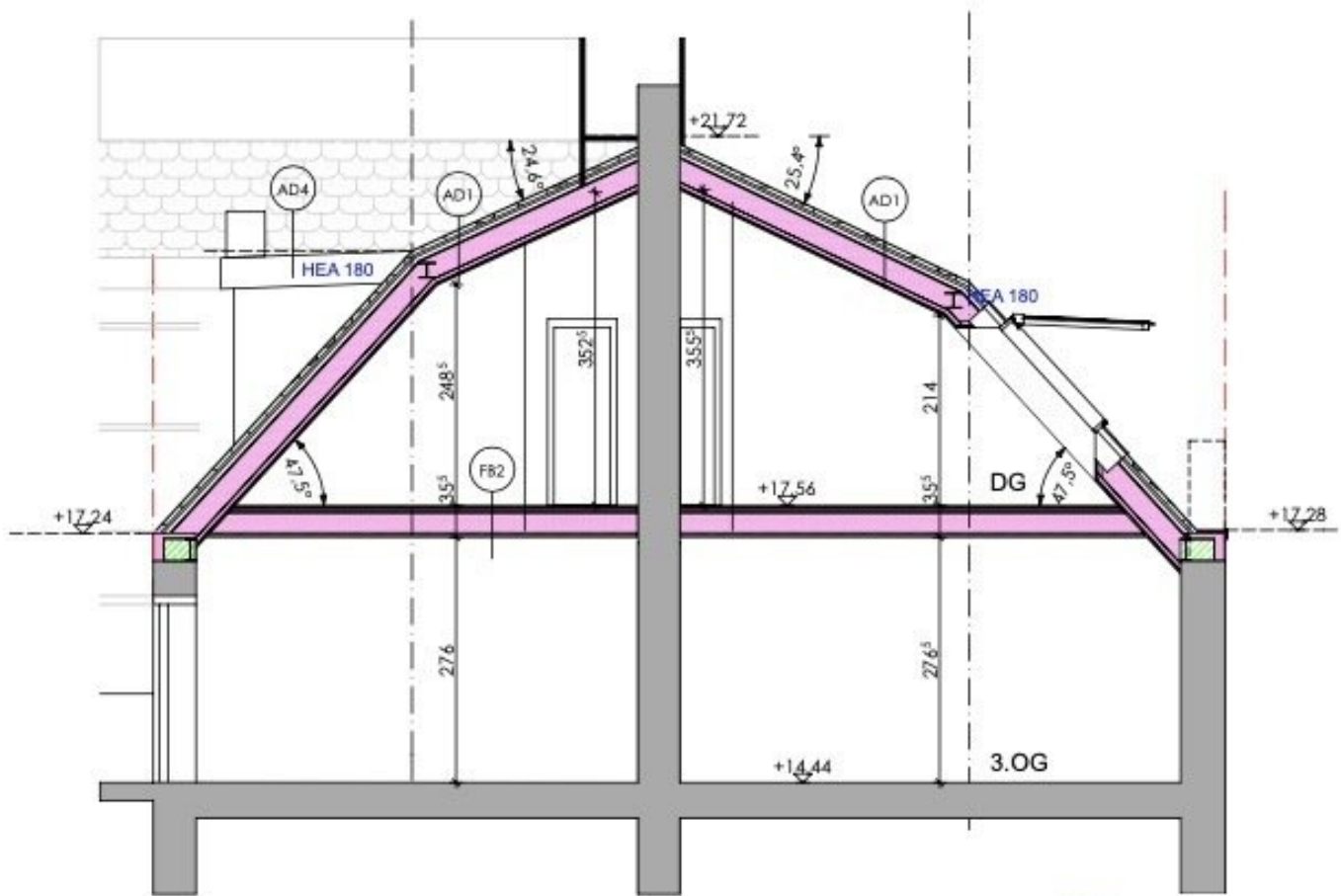
SCHNITT A-A
