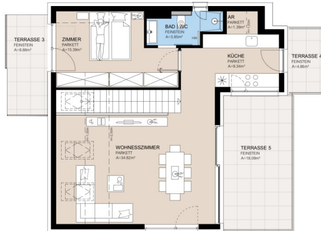
2. DACHGESCHOSS
